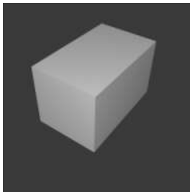
3. Параллелепипед
