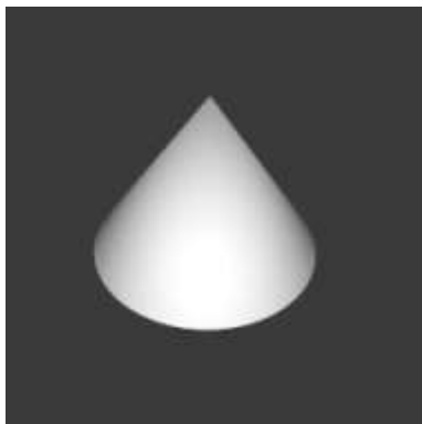
1. Конус
