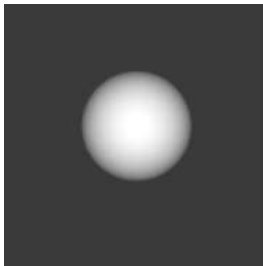
13. Сфера
