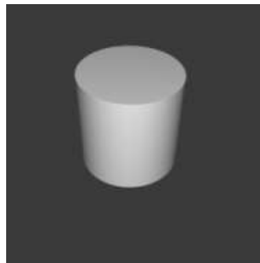
4. Цилиндр
