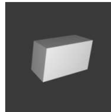
10. Косой параллелепипед
