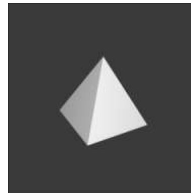
15. Квадратная пирамида
