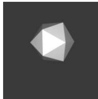
9. Икосаэдр
