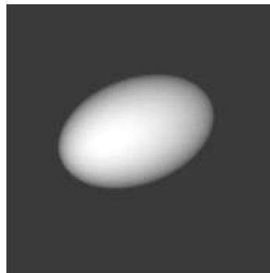
14. Сфероид
